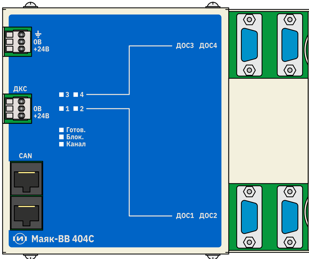
Рисунок А.1 – Внешний вид блока МАЯК-ВВ 404С
