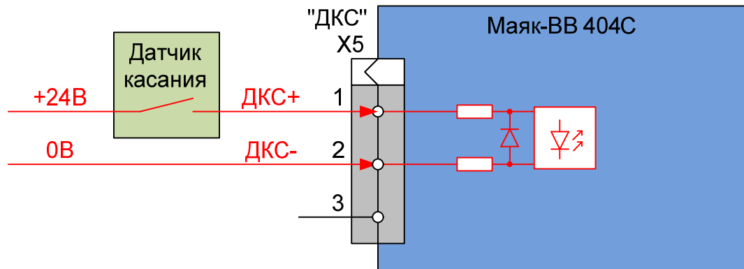
Рисунок Б.3 – Схема подключения датчика касания
