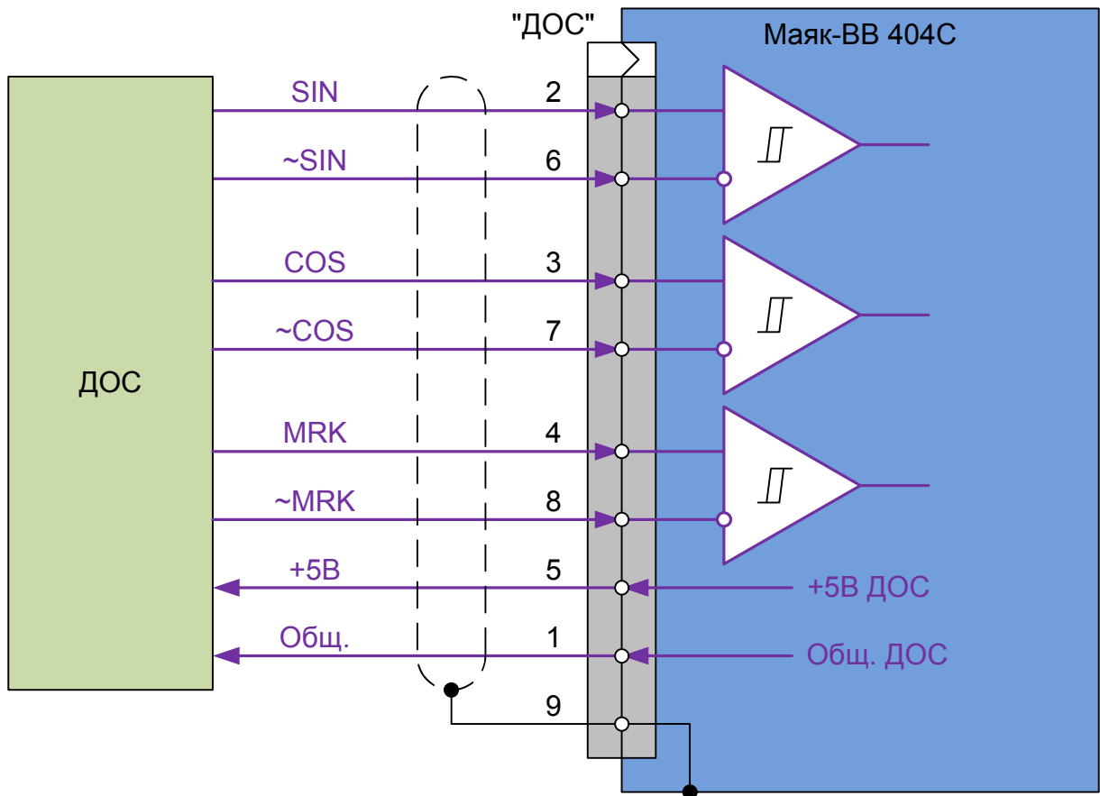
Рисунок А.2 – Схема подключения ДДС
